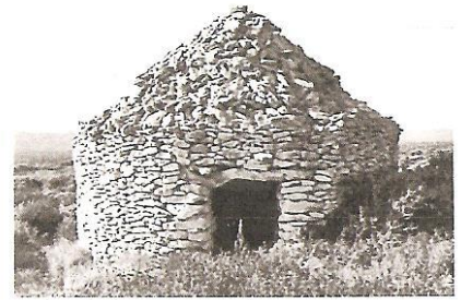
Frankreich: barracun , Korsika
