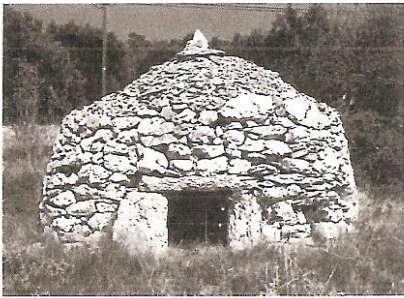
Kroatien: bunja , Festland
