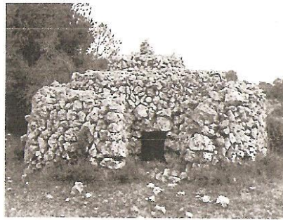
Spanien: Barraca de bestiar , Menorca
