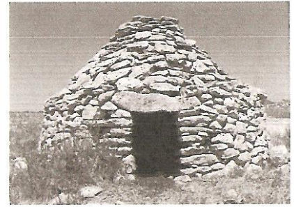
Italien: Pinnetta , Sardinien
